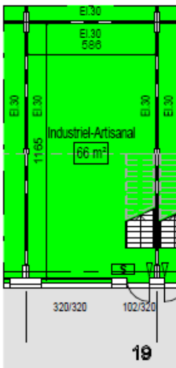
rez-de-chausée C
